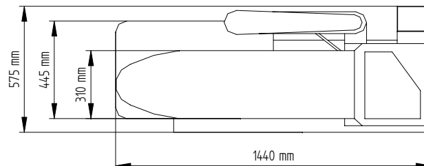
Ansicht von oben / View from the top
