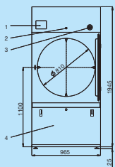
RÜCKANSICHT T 24 35 (DAMPFHEIZUNG)
